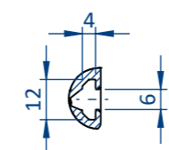
DÉTAIL C ECHELLE 1 : 2 MOUNTING: T-NUT 6MM SLOT, M4
