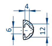
DÉTAIL B ECHELLE 1 : 2 MOUNTING: T-NUT 6MM SLOT, M4
