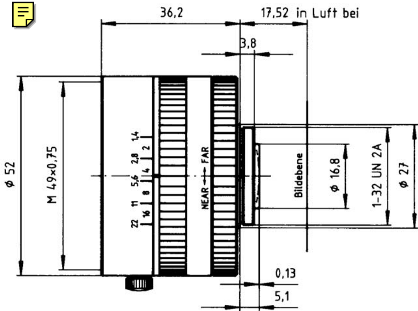
Cinegon 1,4/8 in man. Blendenkörper
