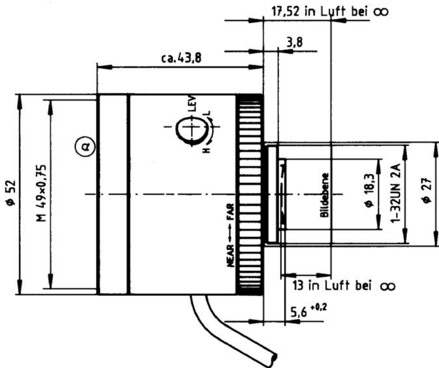
Cinegon 1,4/12 in mot. Blendenregler (VS)
