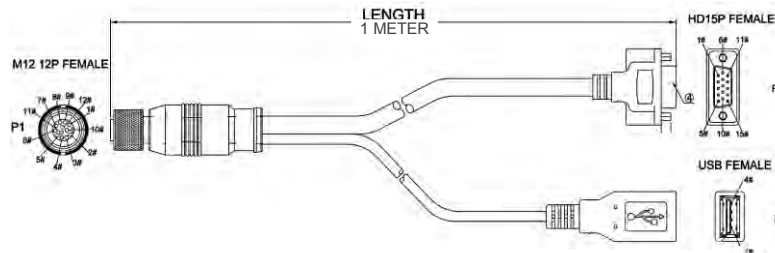
VGA/USB I/O cable P/N: GTR-VGA-USB
